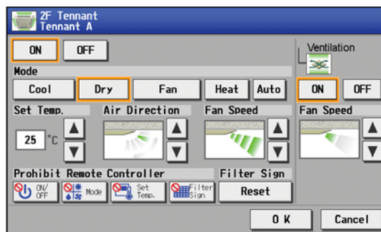
Экран управления блоком системы кондиционирования
